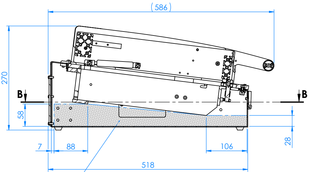
A-A
