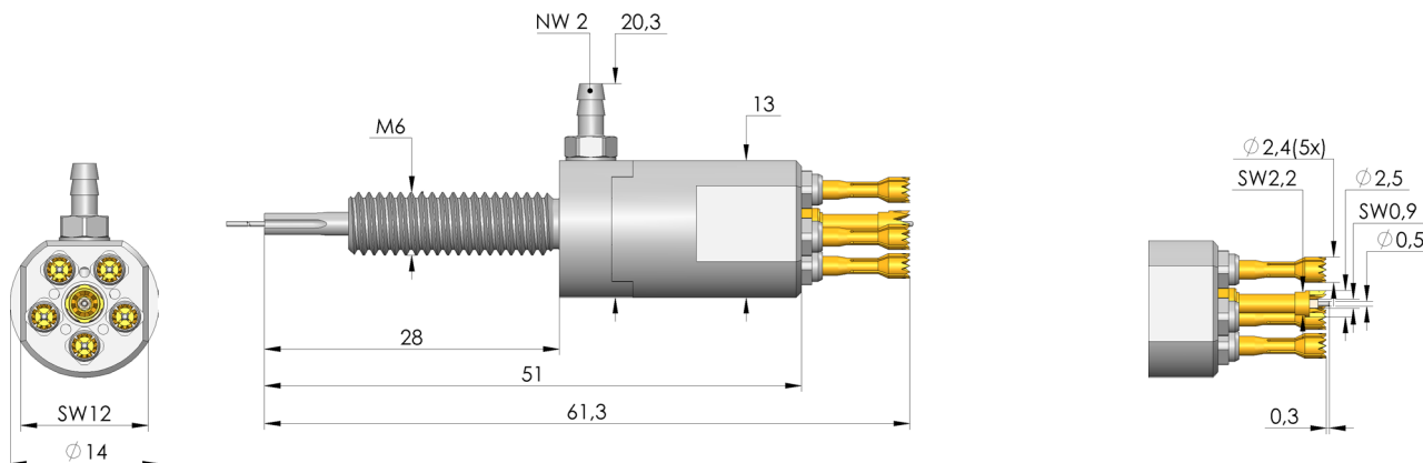
Sense- und Temperaturkontakt TKS-667 388 250 A 5602 M-T5
