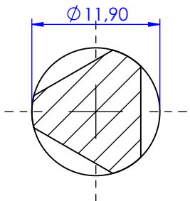
Führungssäule guide pin
