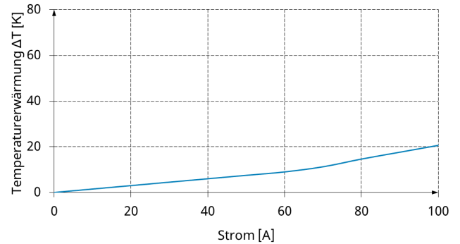
Strombelastbarkeit
