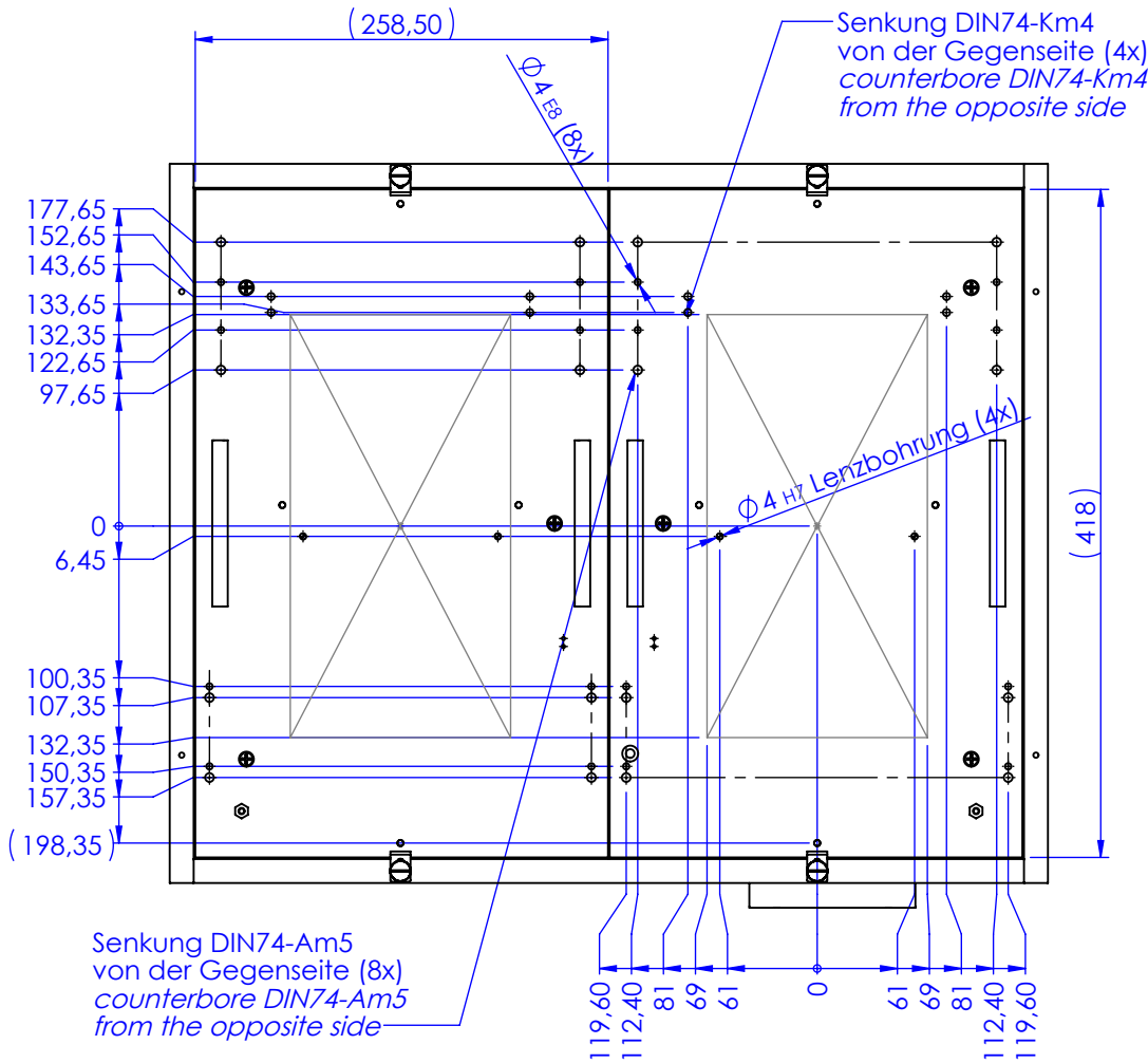
DETAIL X MAßSTAB 1 : 2
