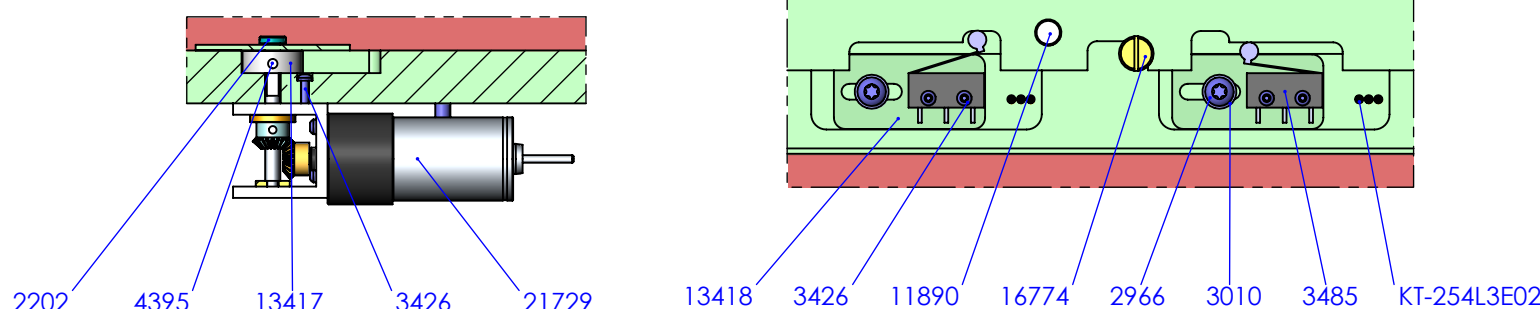
DETAIL X MAßSTAB 1 : 2
