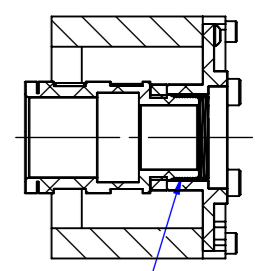
SCHNITT B-B MABSTAB 1 : 2
