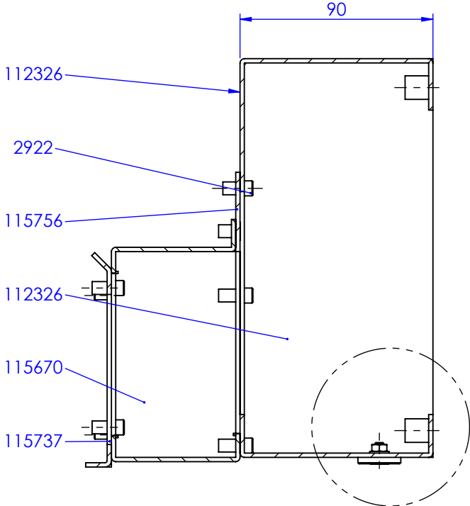
SCHNITT A-A MAßSTAB 1 : 2.5
