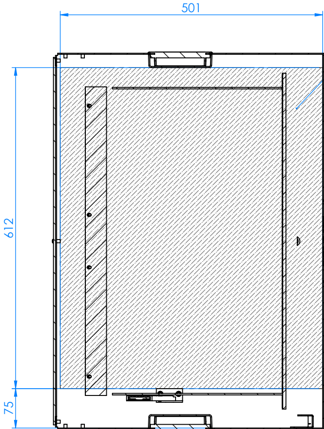
B-B
