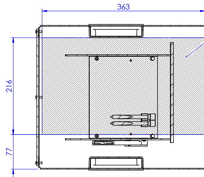
B-B
