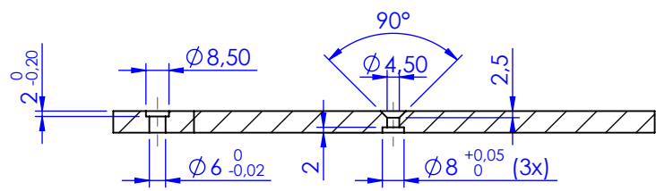
SCHNITT A-A
