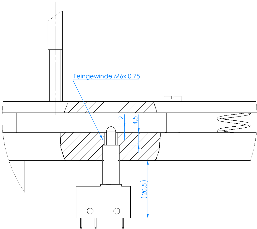
DETAIL A MAßSTAB 1.5 : 1
