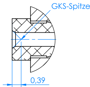
DETAIL A MAßSTAB 10 : 1
